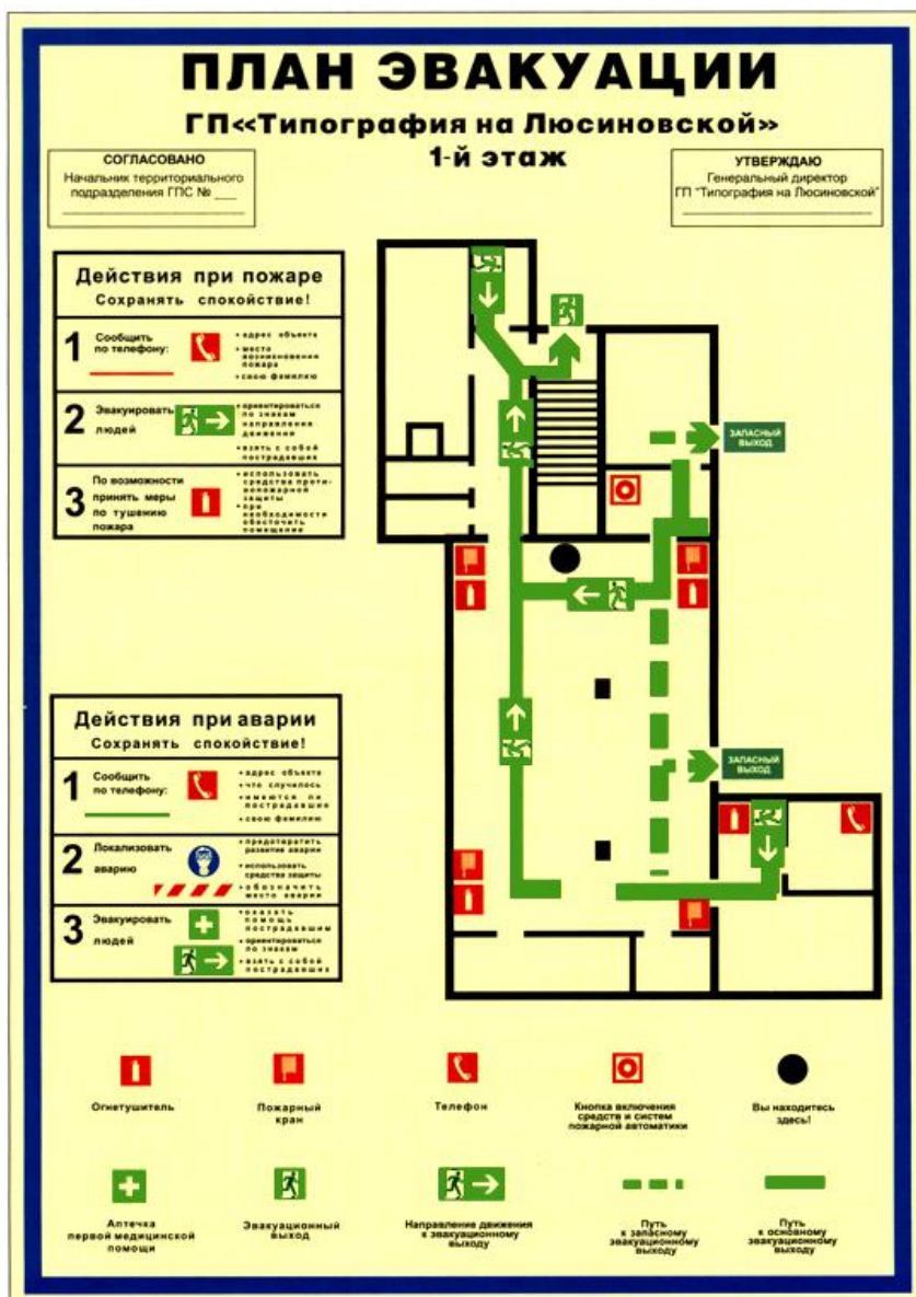
Рисунок В.1 - Этажный план эвакуации (фотолюминесцентный)
