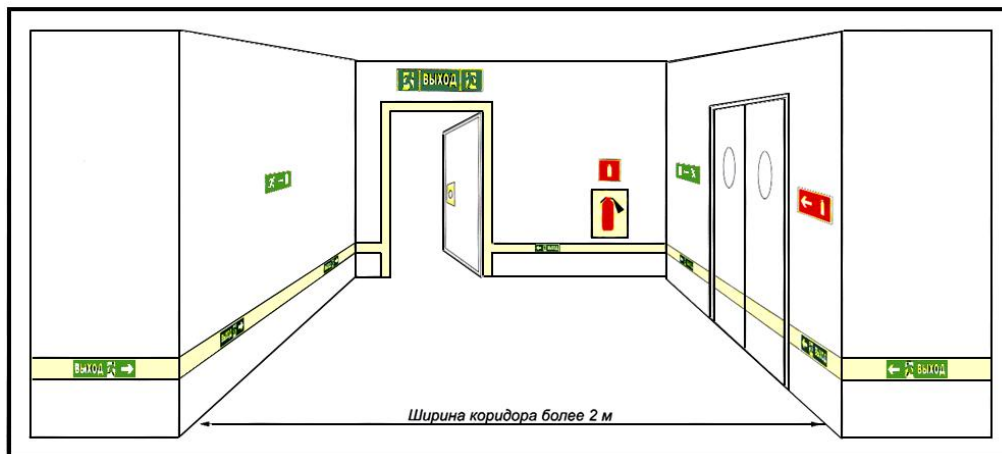
Рисунок Б.2 - Пример обозначения элементами ФЭС коридора.
