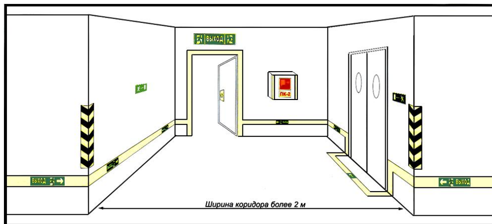
Рисунок Б.1 - Пример обозначения элементами ФЭС коридора.
