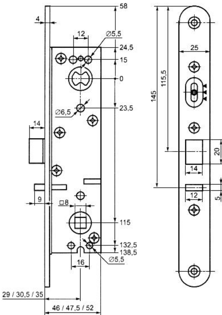
Рисунок А.5 - Пример замка электромеханического бесключевого устройства "Антипаника" для дверей эвакуационных выходов
